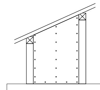
妻パネル
